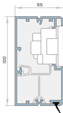
Przekrój kanału MC 100/55 A.
