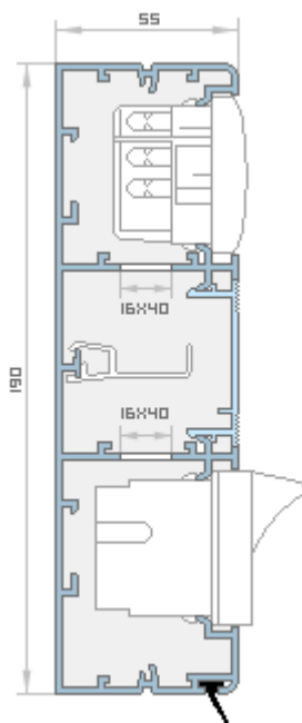
Przekrój kanału MC 190/55 A.
