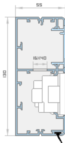
Przekrój kanału MC 130/55 A.
