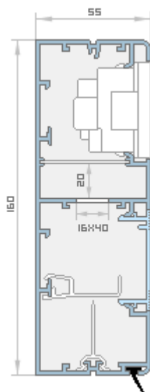
Przekrój kanału MC 160/55 A.
