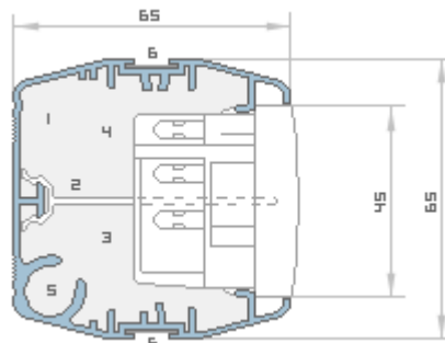
Przekrój poprzez słupek CODI MC 65/65 .
