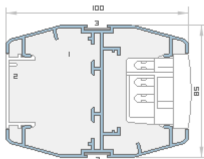
Przekrój słupka CODI MC 110/80.
