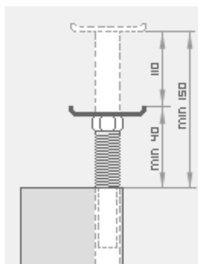
Widok sztycy rozporowej, mocującej słupek od strony sufitu.
