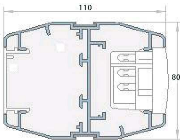
Przekrój popularnego słupka Codi MC 110/80.
