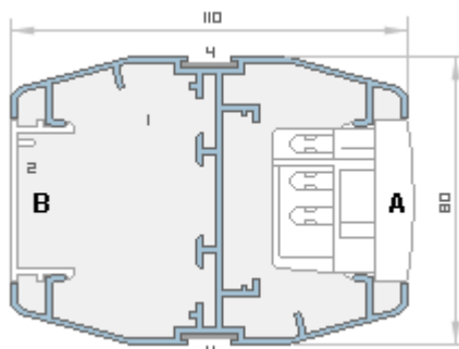
Przekrój kolumnienki CODI MC 110/80.
