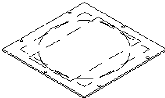
Szkic ramy montażowej UDM2 (różne otwory pod pokrywy).
