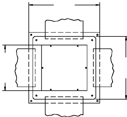
Widok z góry puszek podłogowej UDH.
